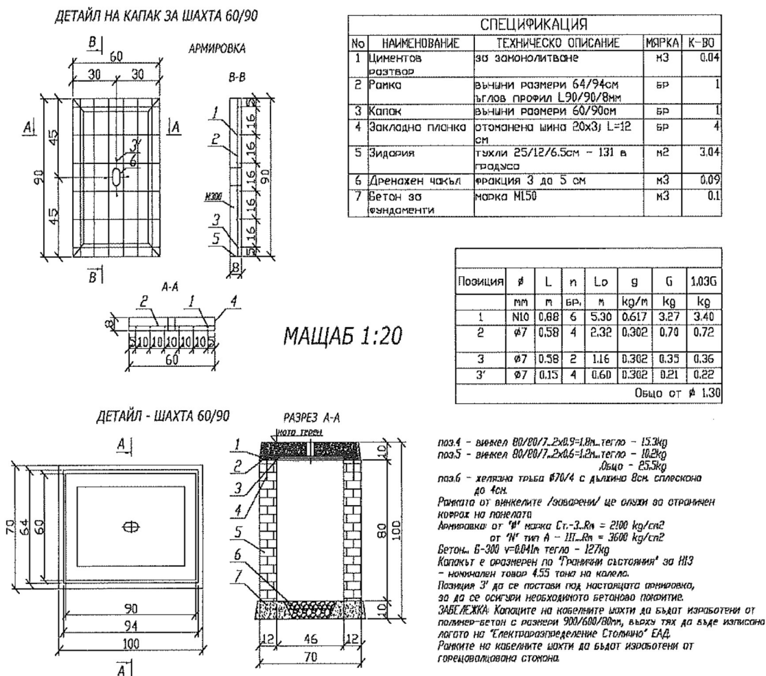
Фиг. 6.3. Кабелна шахта – единична
